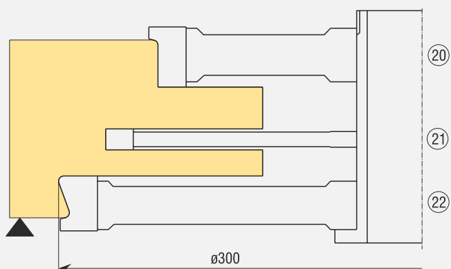
F doprozornik: vertikala gore
