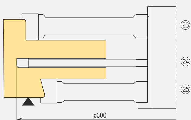
G doprozornik: vertikala dolje
