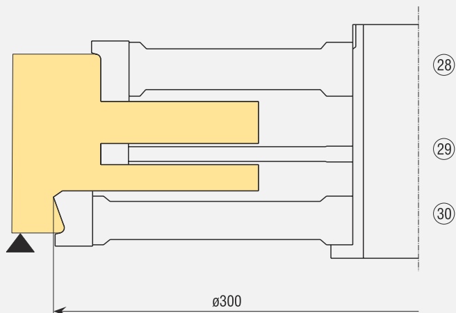
J krilo: čep
