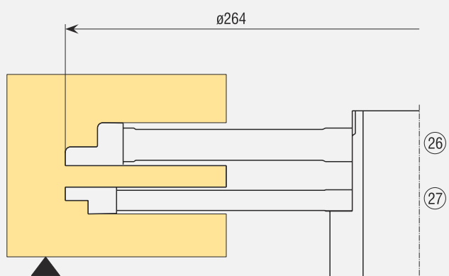
H doprozornik: horizontala
